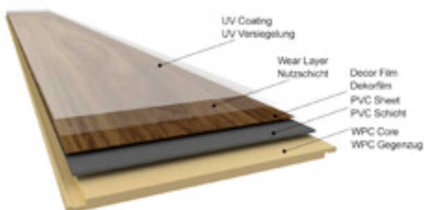
Aufbau WSL Diele Structure WSL Plank 5.5/0.3mm
